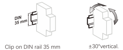
Clip on DIN rail 35 mm
