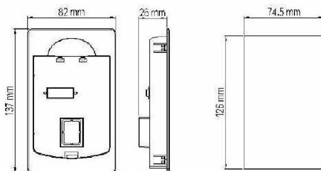
Выносная панель управления и установочные размеры
